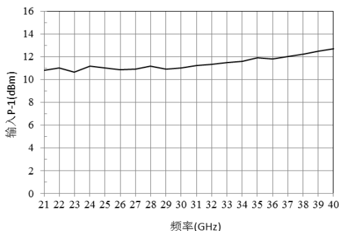
输入 P-1@LO=13dBm
