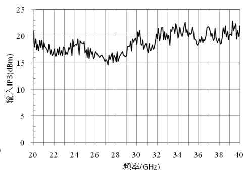
输入 IP3@LO=13dBm
